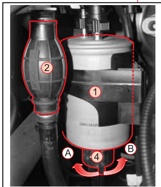
Топливный фильтр
