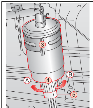
Водоотделитель
